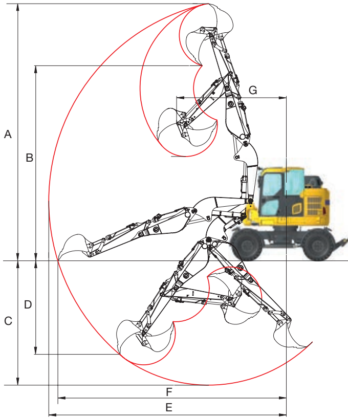
Diagramma di scavo
